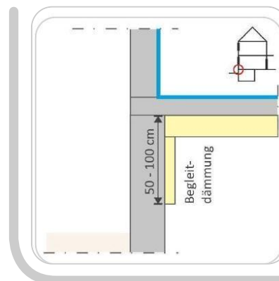
Begleitdämmung
